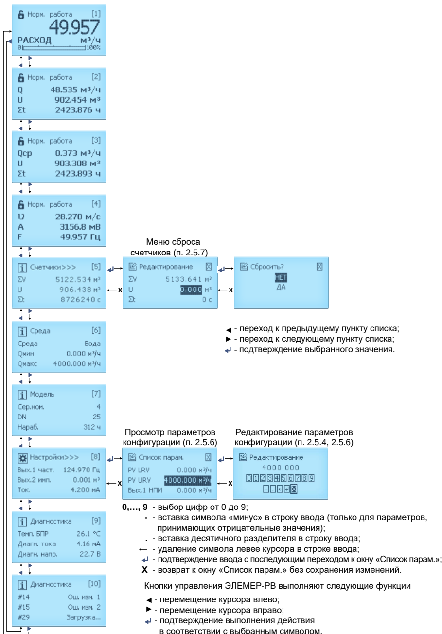
Рисунок 2.11 – Меню ЭЛЕМЕР-РВ
